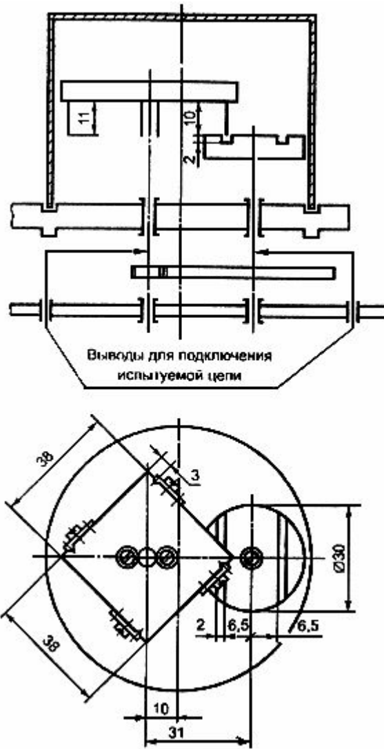
Рисунок 2 - Кинематическая схема искрообразующего механизма I типа
