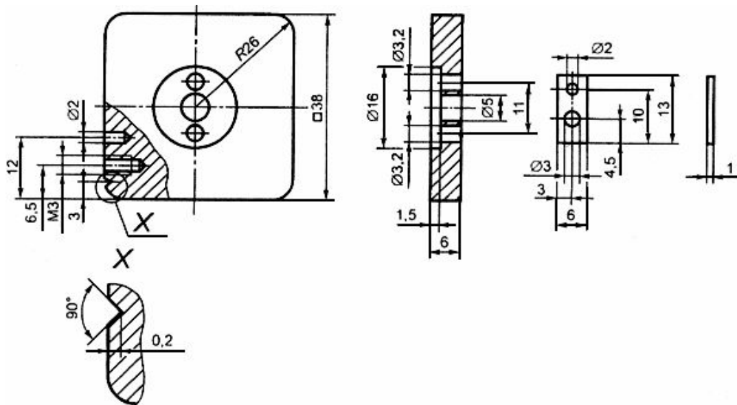
Рисунок 4 - Держатель провололочек
