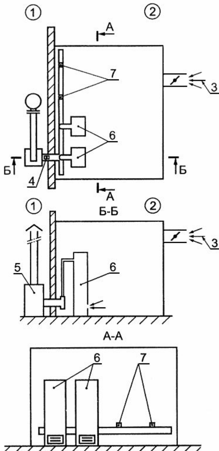
1 - взрывоопасная зона; 2 - взрывобезопасная зона; 3 - вход воздуха; 4 - датчик расхода; 5 - вентиляционное оборудование; 6 - кожуха анализаторов, соединенные с вентиляционными коробами; 7 - запасные соединения для дополнительных анализаторов Рисунок С.1
